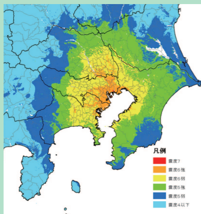
平成25年12月19日公表の首都直下地震の想定 (被害量推計に用いた震度分布図)
